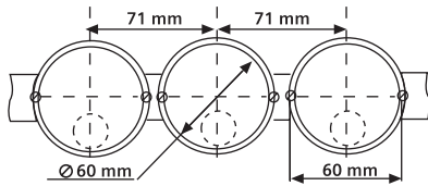
Duvar içi montaj ölçüsü
